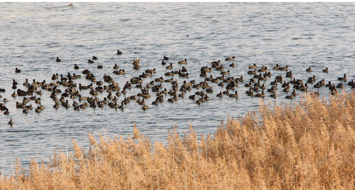
Lyski na jeziorze Wigry na wysokości punktu widokowego w Bryzglu KORMORANÓW PIĘĆ RAZY MNIEJ
