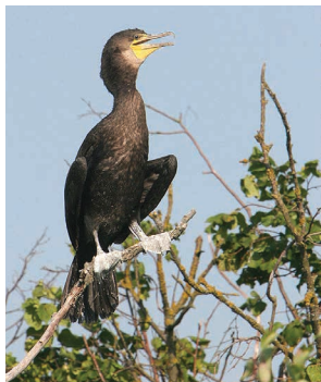
Dorosły kormorana zjada ponad pół kilograma ryb dziennie
